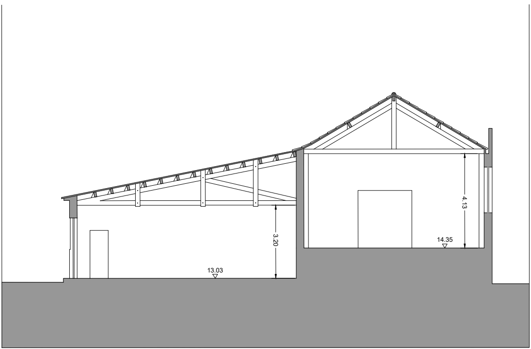
CORTE T3
