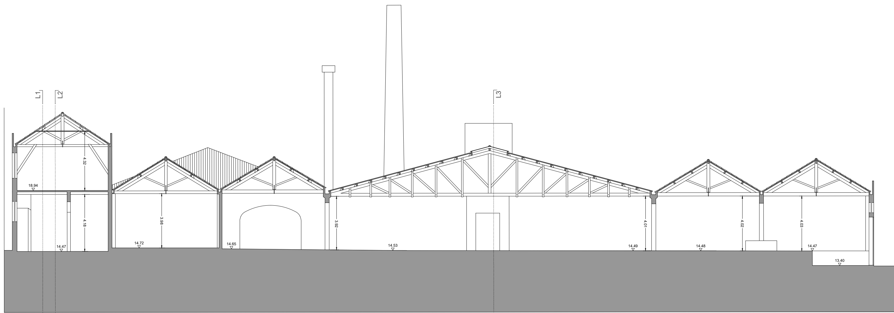
CORTE T2
