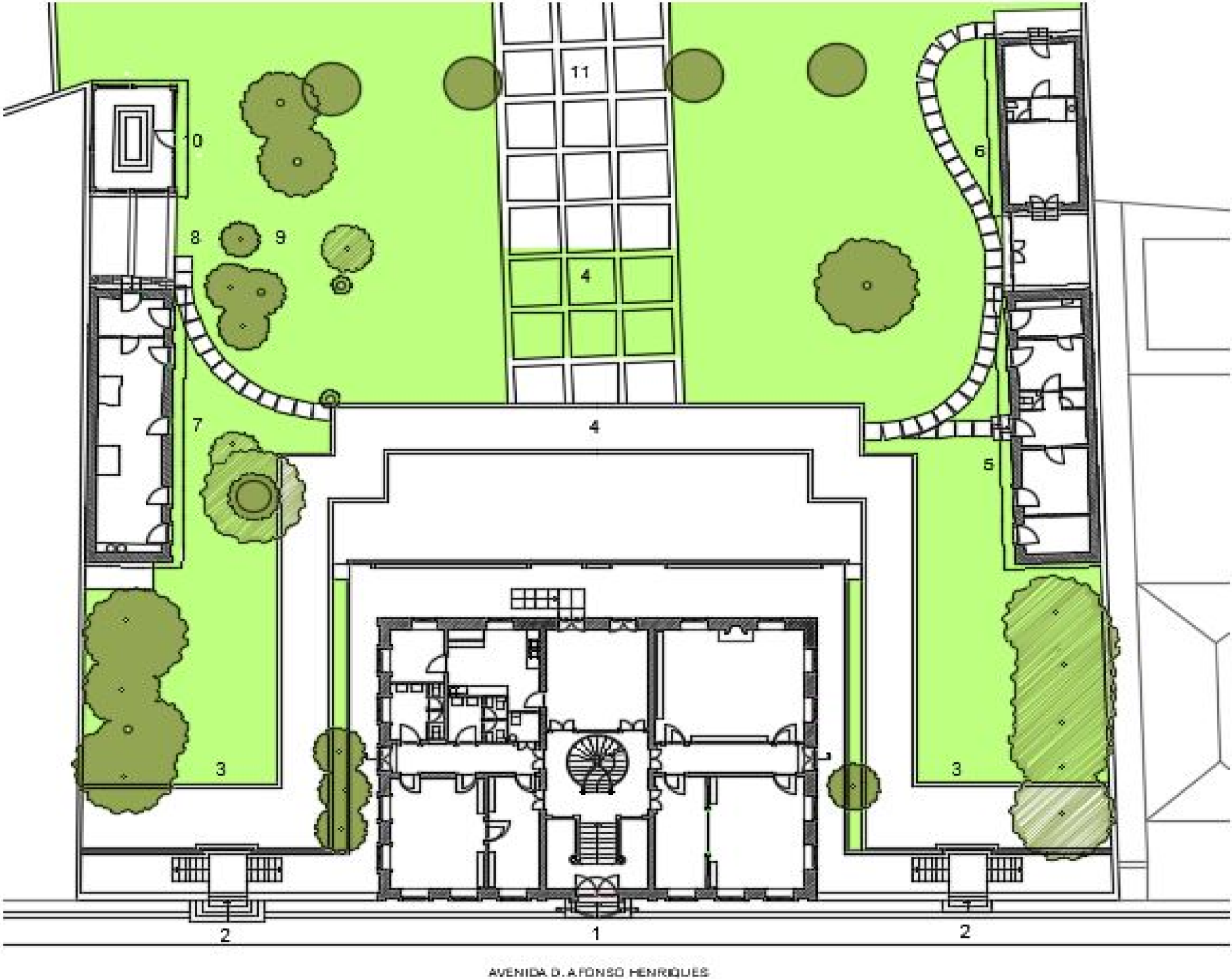
Planta de Enquadramento
