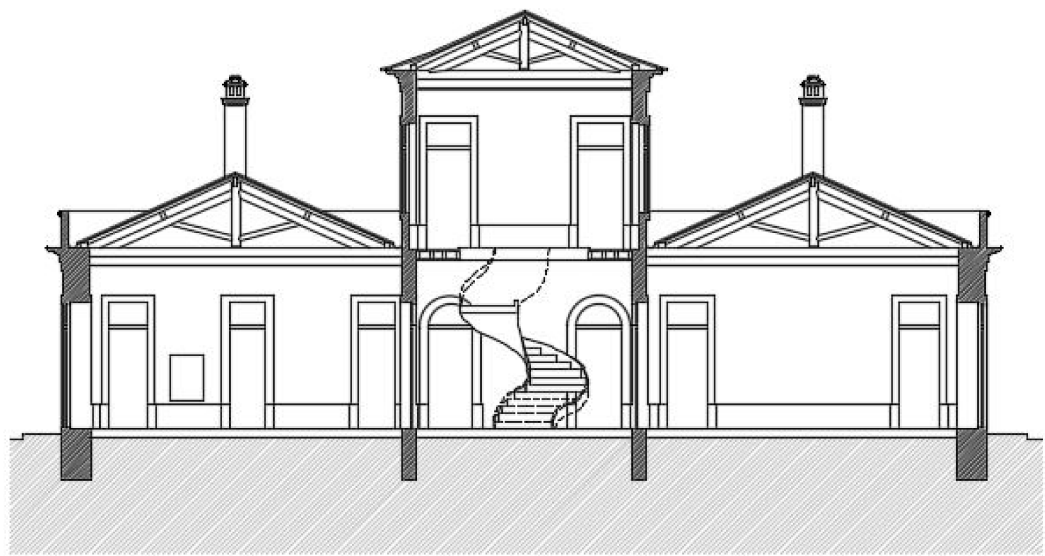
CORTE AB
