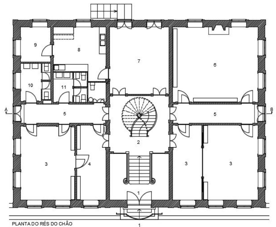
Planta do Rés do Chão
