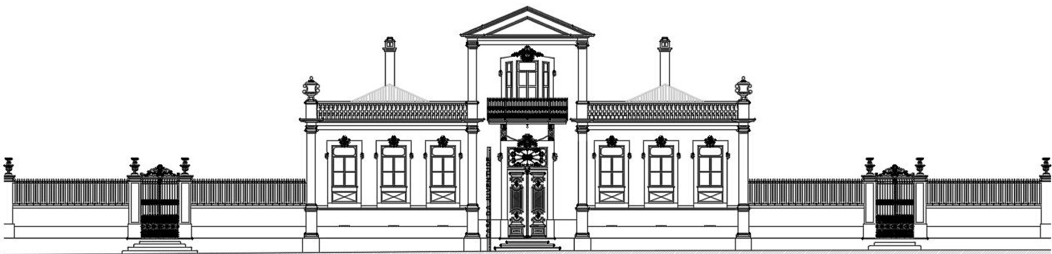
ALÇADO POENTE
